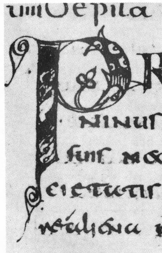
d: Par. lat. 13028 Bl. 65' nach Zimmermann, Vorkarol. Min. Tafel 115 c
